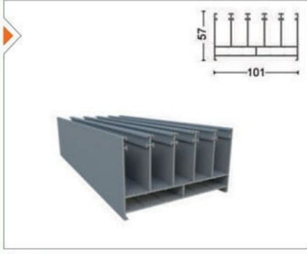
SRM-1001 Üst Kasa Profili Upper Frame Profile
