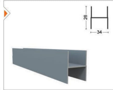
YNSRM-1009 Birleştirme Adaptörü Joining Adapter
