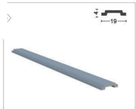
ISICM31-1013 Tij Profili Ağırılık/Weight Push Rod Profile 0.123 kg/m
