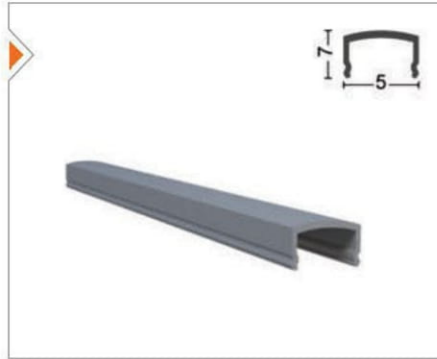
GYTN-1504 Küpeşte Çıtası Profili Railing Slot Profile
