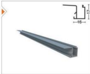
AD-1008 Aldoks İsicam Çıtası Aldox Bead Profile For Double Glass
