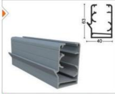
GLD-1002 Oluklu Kasa Profili Dropper Frame Profile
