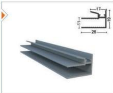
SRM-1010 Çekme Profili 8 mm Pull Profile 8 mm
