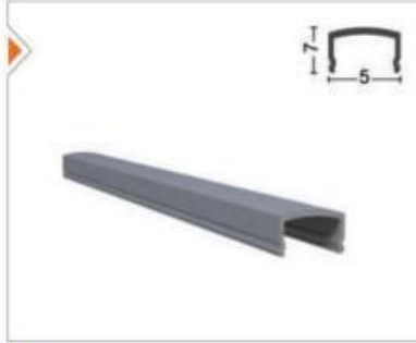
GYTN-1504 Küpeste Çıtası Profili Railing Slot Profile
