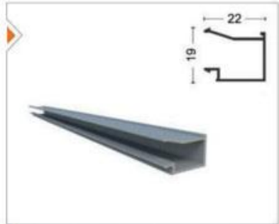
C60-1006 C-60 İsicam Çıtası C-60 Bead For Double Glass Profile
