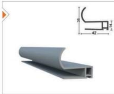
SRM-1008 Sürme Bitim Profili End Profile
