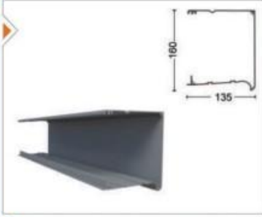
GYTN-1501 Üst Kutu Profili Upper Box Profile
