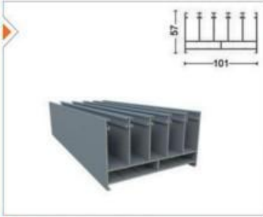
SRM-1001 Üst Kasa Profili Upper Frame Profile
