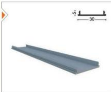
YNSRM-1010 Dikme Kapama Çıtası Side Cover Profile
