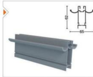
YNSRM-1006 Bitim Profili End Profile
