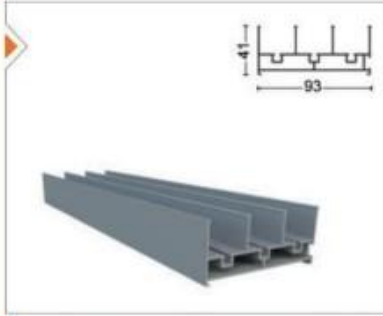
YNSRM-1001 Kasa Profili Frame Profile
