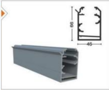
PRGLD-1001 Oluklu Kasa Profili Dropper Frame Profile
