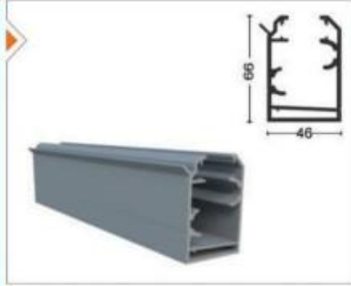
PRGLD-1001 Dökme Kasa Profili Dropper Frame Profile
