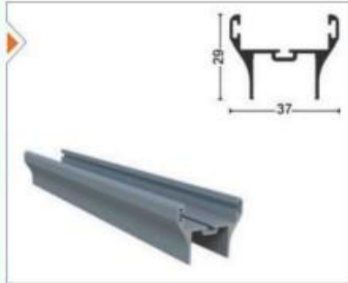
ISiCM21-1005 Büyük H Fıtil Big "H" Aluminum Seal
