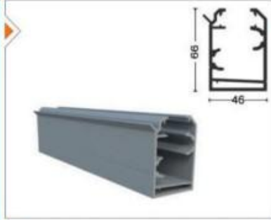
PRGLD-1001 Dökümlü Kasa Profili Dropper Frame Profile
